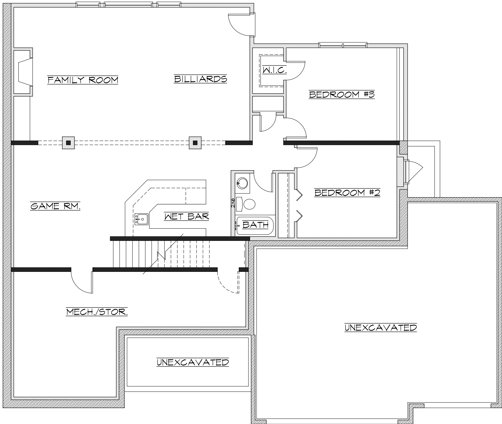
LOWER FLOOR PLAN N.T.S.
